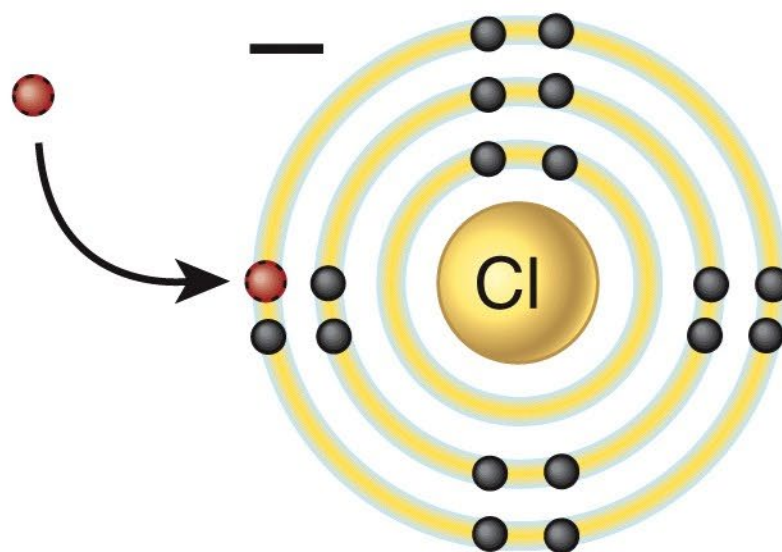
Ion
